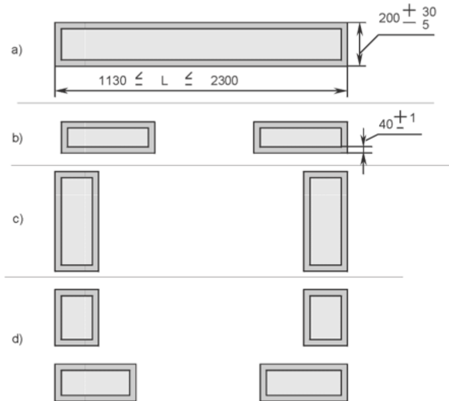
Joonis 3. Haagise tunnusmärk
