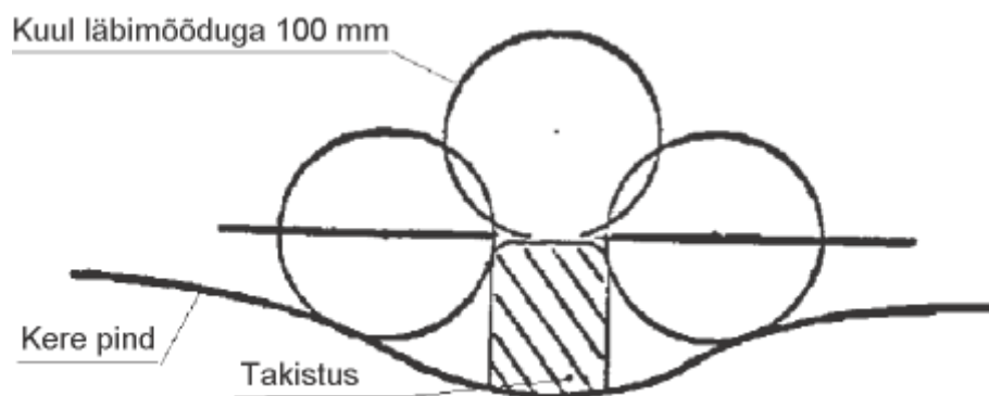
Joonis 14. \emptyset 100 mm kuuli veeretamine üle kere pinnal olevast takistusest
