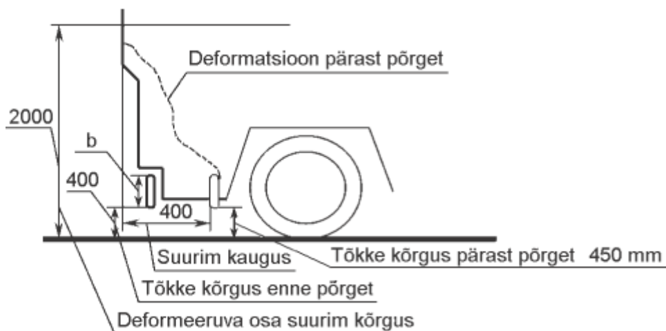
Joonis 19. Tõkke külgvaates. Lubatud deformatsioonid. b – tõkke profiili laius
