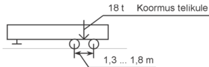
Joonis 46. Tandemtelgede asetus
