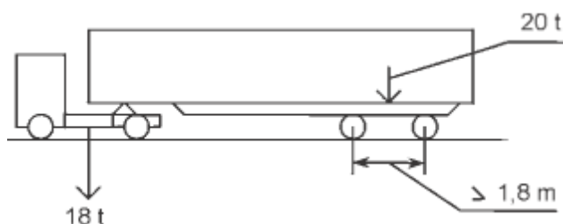
Joonis 47. Autorongi koormus ja poolhaagise tandemtelgede asetus
