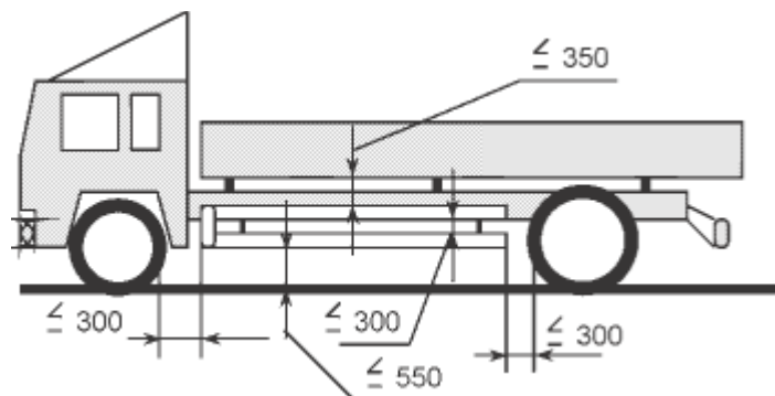
Joonis 20. Külgmise allasõidutõkke asukoht mootorsõidukil
