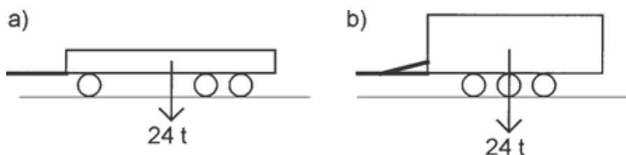
Joonis 44. a) täishaagis; b) kesktelghaagis
