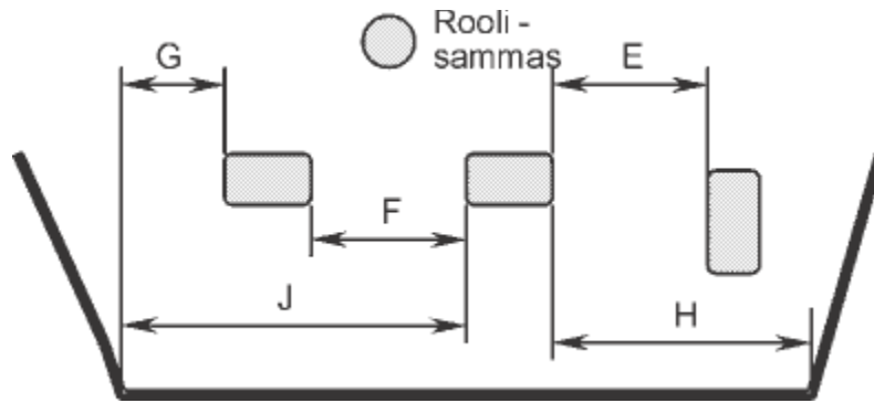
A. Kolme pedaali asend. Mõõtmised on toodud tabelis 6
