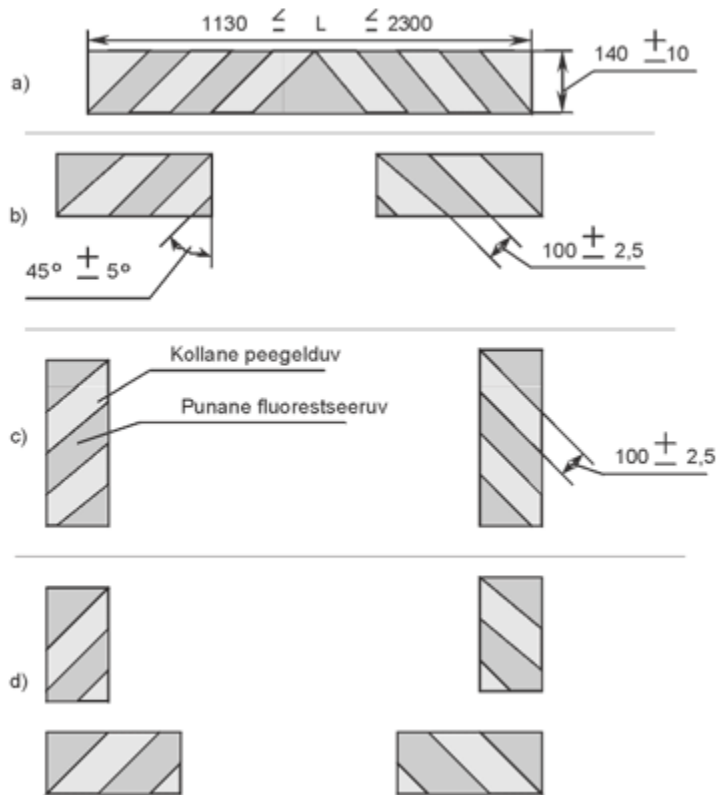
Joonis 4. N 3 kategooria sõiduki tunnusmärk
