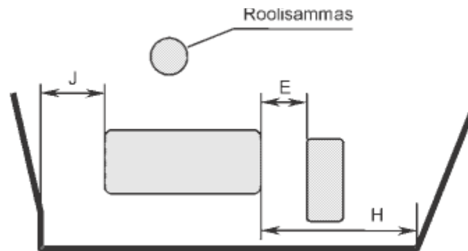
B. Kahe pedaali asend. Mõõtmised on toodud tabelis 7
